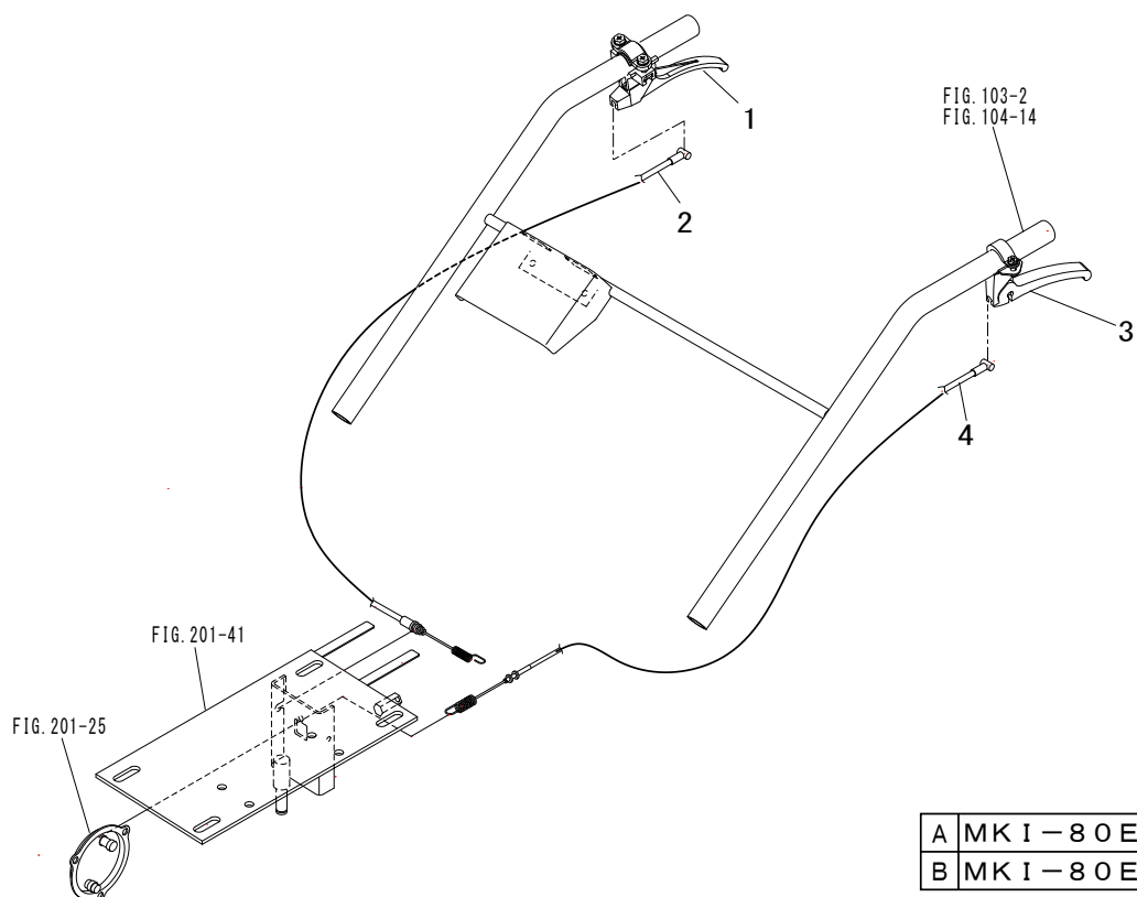
FIG. 302 クラッチ レバー
