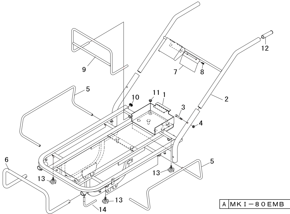
FIG.103 メイン フレーム 1
