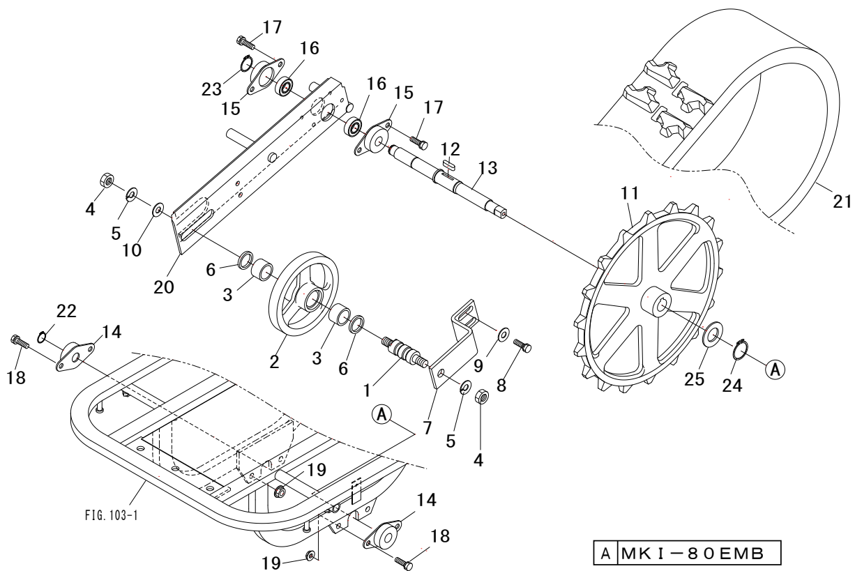
FIG. 101 クローラ フレーム 1
