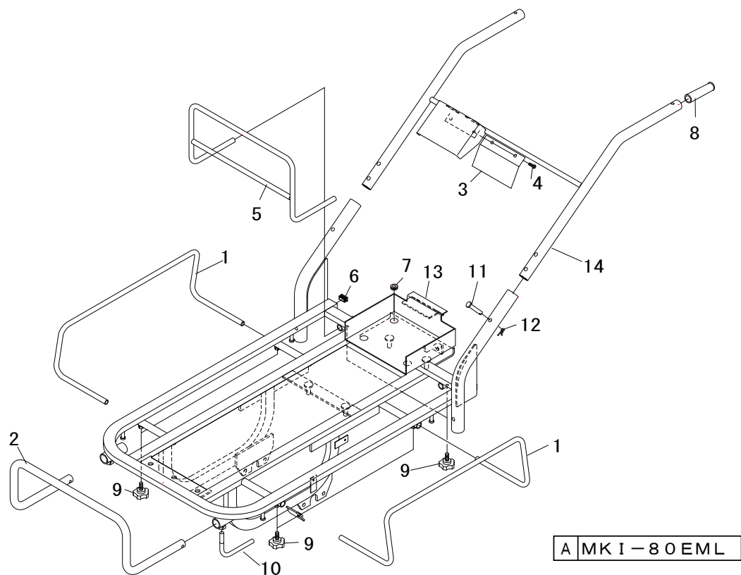
FIG.104 メイン フレーム 2
